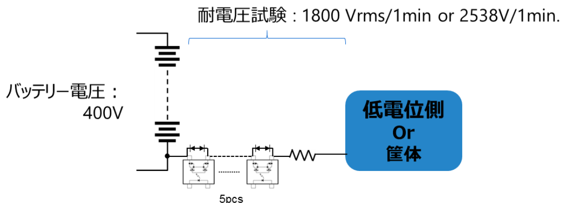
図 8 地絡検出回路 (バッテリー電圧 : 400V)
