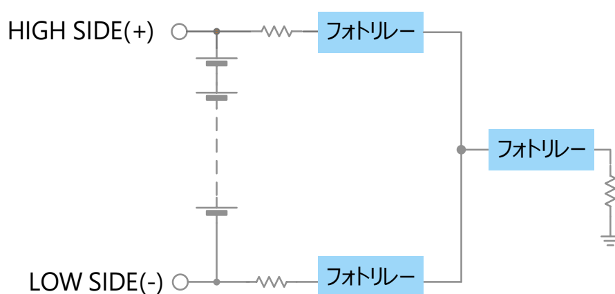
図6 地絡検出回路 (例)
