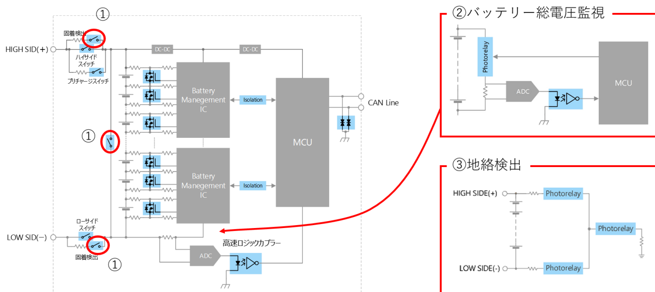
図 3 高耐圧フォトリレー応用ブロック図
