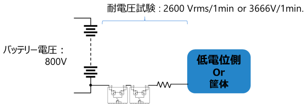
図 7 地絡検出回路 (バッテリー電圧 : 800V)
