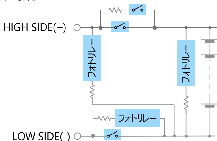
図 4 メカリレー溶着検知回路 (例)
