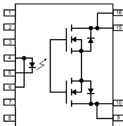
(b) TLX9160T 内部構造図
