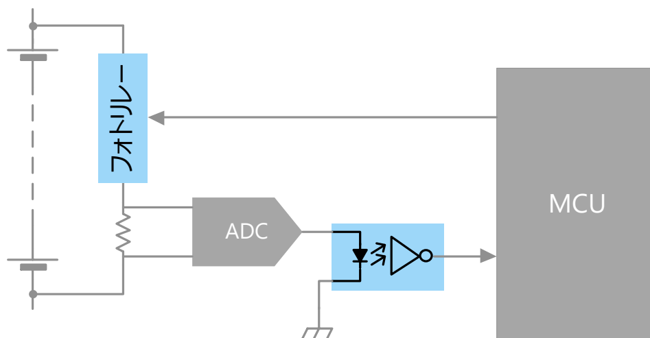
図5 バッテリー総電圧監視回路 (例)
