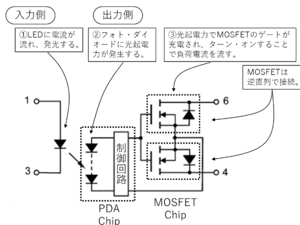
図 2(a) フォトリレー動作原理
