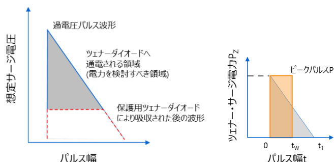
図 3.3 サージ波形から方形波近似しパルス幅の導出例
