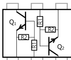
c) 点対称タイプ
