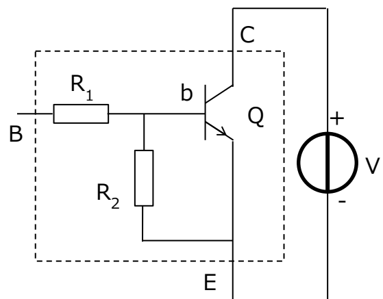
図 4-2 I_{CEO}
