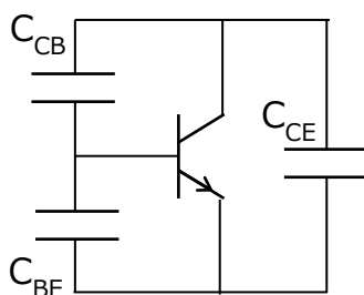
図 4-9 トランジスターの容量
