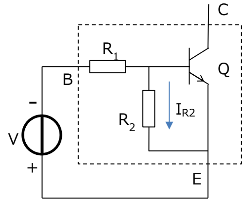
図 4-3 I_{EBO}
