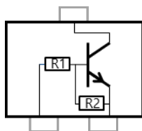
a) シングル
