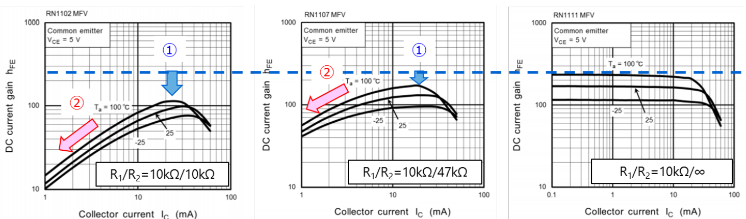
図 4-5 h_{FE} と R_2 の関係
