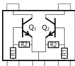
b) エミッタコモンタイプ
