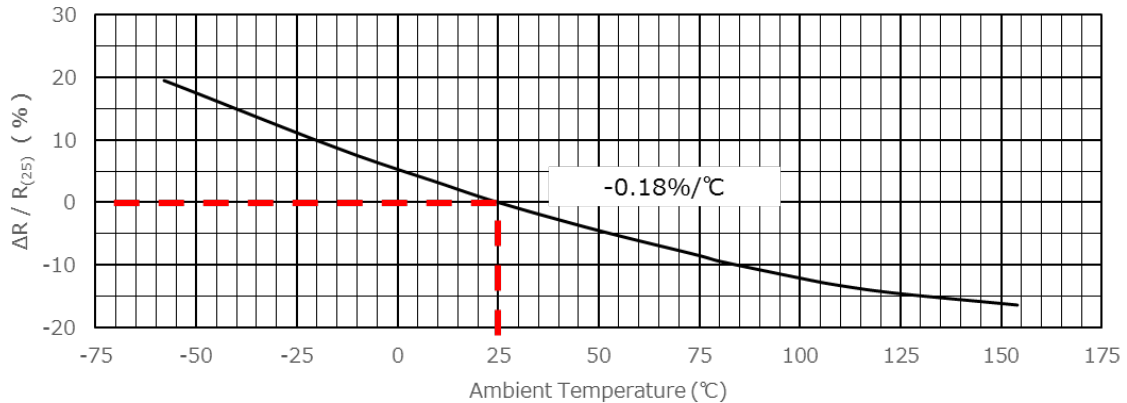
図 4-11 内蔵抵抗温度特性例（25℃基準）
