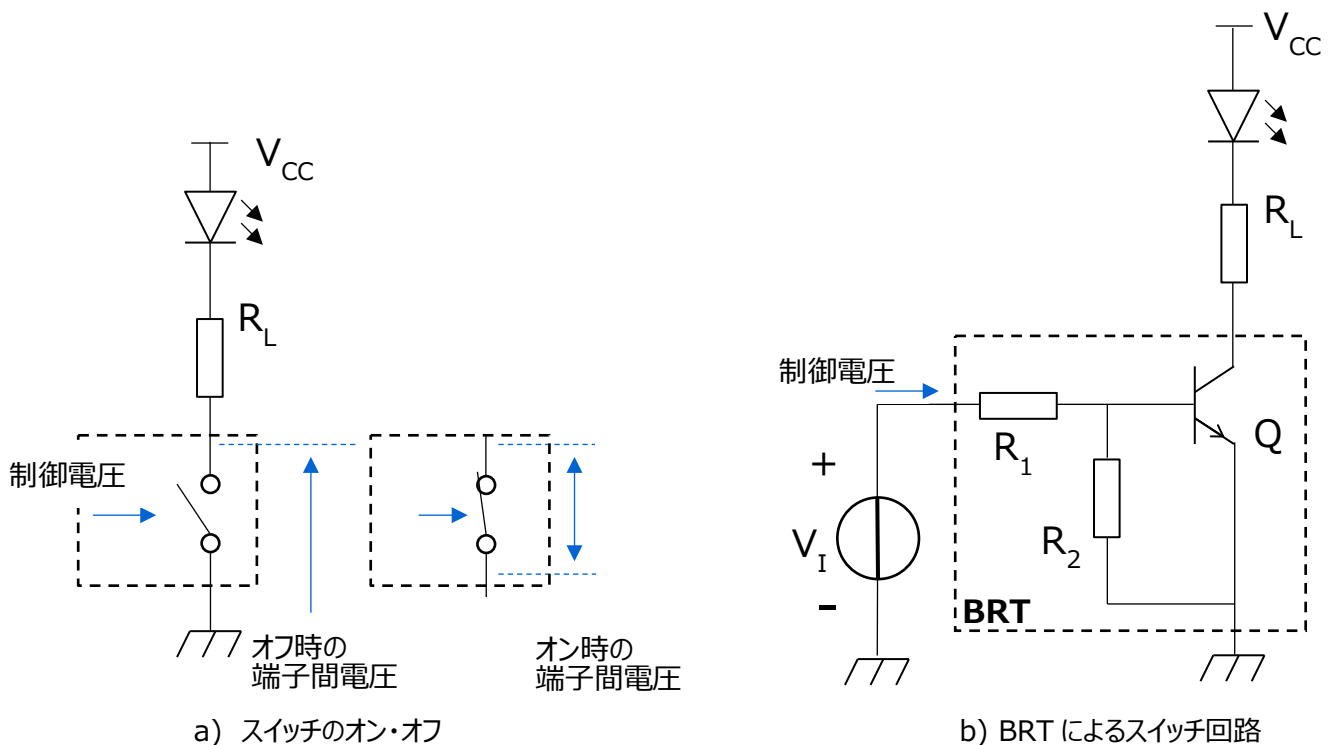
図 1-1 スwitchのオン・オフ と BRT によるスイッチ回路
