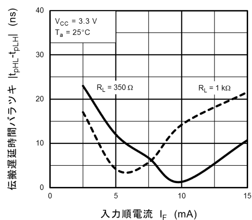
図 12.2.22 |t_{pHL} - t_{pLH}| - I_F
