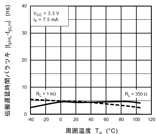
図 12.2.16 |t_{pHL} - t_{pLH}| - T_a
