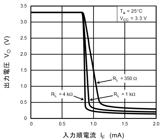
図 12.2.7 V_O - I_F
