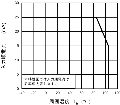
図 12.2.2 I_F - T_a
