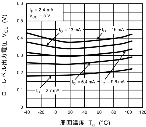
図 12.2.4 V_{OL} - T_a
