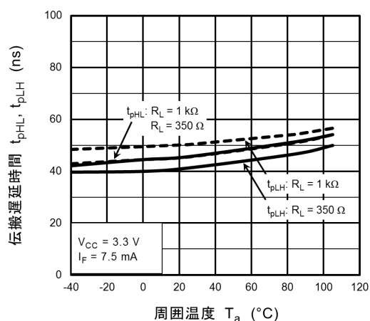
図 12.2.15 t_{pHL}, t_{pLH} - T_a
