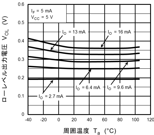
図 12.2.6 V_{OL} - T_a
