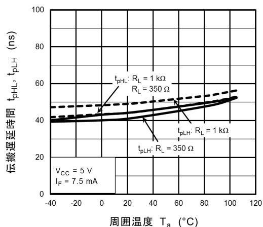
図 12.2.19 t_{pHL}, t_{pLH} - T_a
