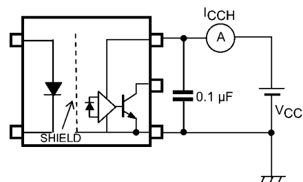
図 12.1.4 I_{CCH} 測定回路
