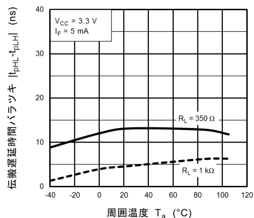
図 12.2.14 |t_{pHL} - t_{pLH}| - T_a
