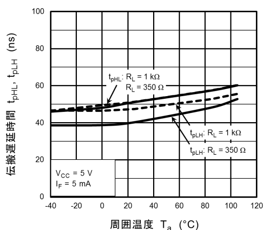
図 12.2.17 t_{pHL}, t_{pLH} - T_a
