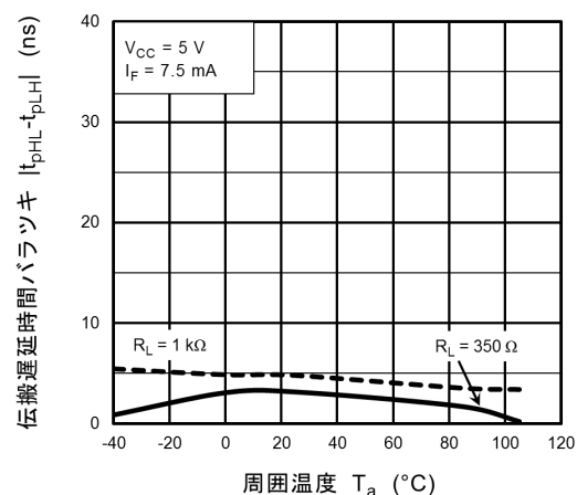
図 12.2.20 |t_{pHL} - t_{pLH}| - T_a
