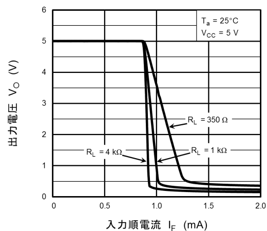
図 12.2.8 V_O - I_F
