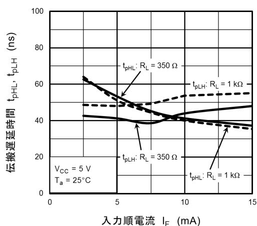
図 12.2.23 t_{pHL}, t_{pLH} - I_F
