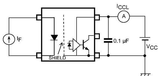
図 12.1.3 I_{CCL} 測定回路
