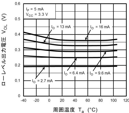
図 12.2.5 V_{OL} - T_a
