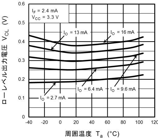
図 12.2.3 V_{OL} - T_a
