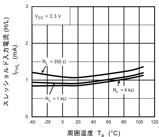
図 12.2.9 I_{FHL} - T_a
