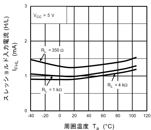
図 12.2.10 I_{FHL} - T_a
