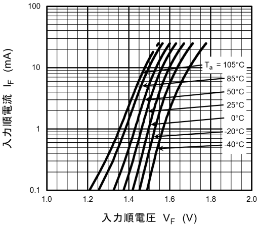
図 12.2.1 I_F - V_F
