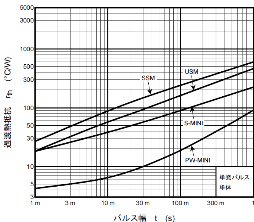
図 1.6 パッケージ別 r_{th} - t 特性例
