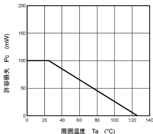
図 1.5 スモールスーパーミニ, ウルトラスーパーミニ許容損失 P_c -周囲温度 T_a
