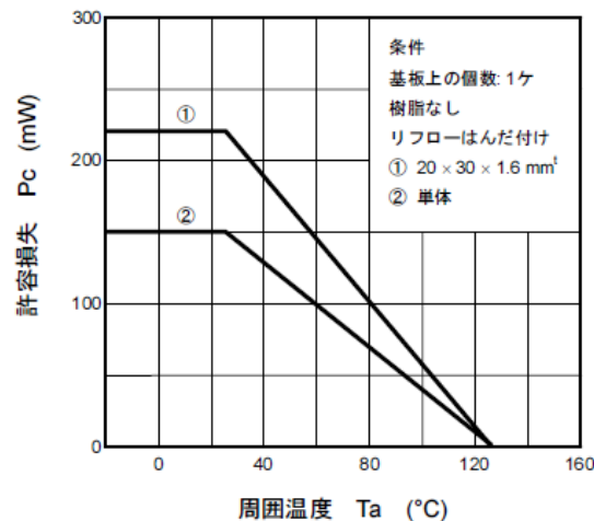
図 1.2 エポキシガラス基板取り付け時の P_C-T_a 特性
