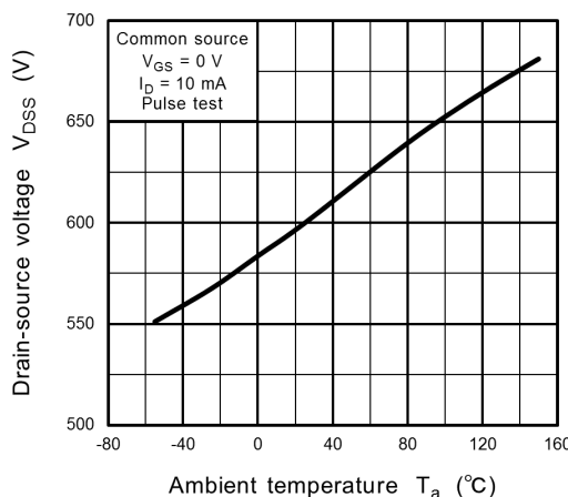
Fig. 8.5 V_{DS} - T_a
