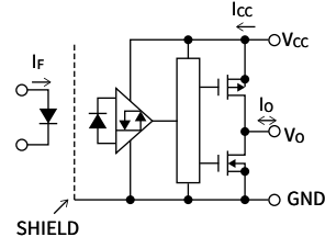
Totem-Pole Output
