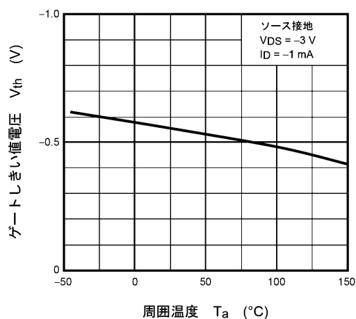
図 8.7 V_{th} - T_a
