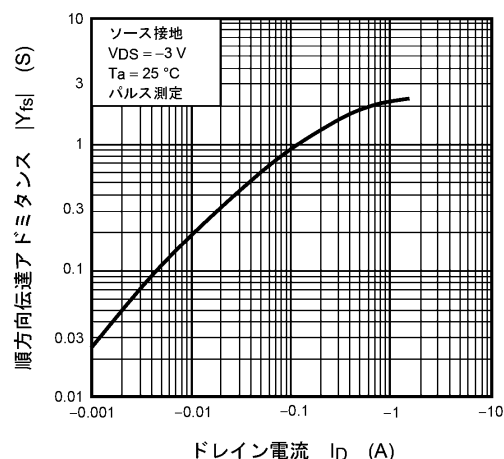
図 8.8 |Y_{fs}| - I_D
