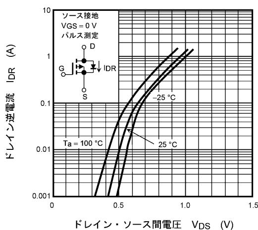
図 8.9 I_{DR} - V_{DS}
