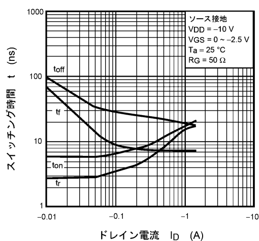
図 8.11 t - I_D
