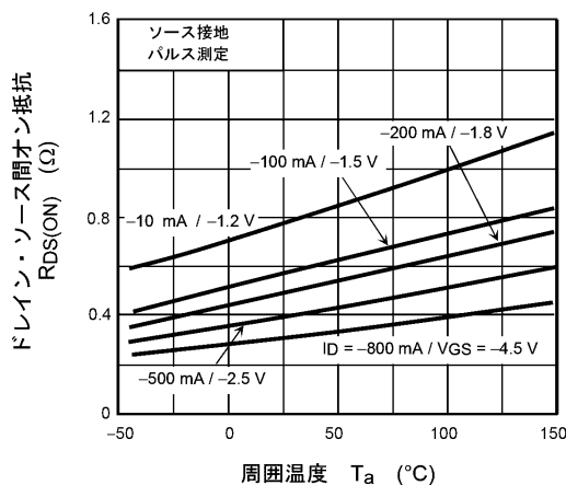
図 8.6 R_{DS(ON)} - T_a
