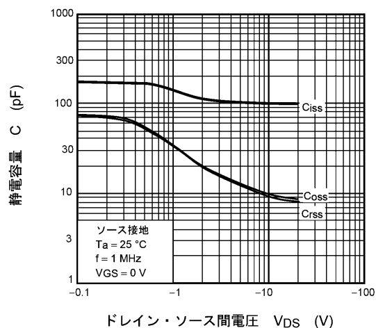
図 8.10 C - V_{DS}
