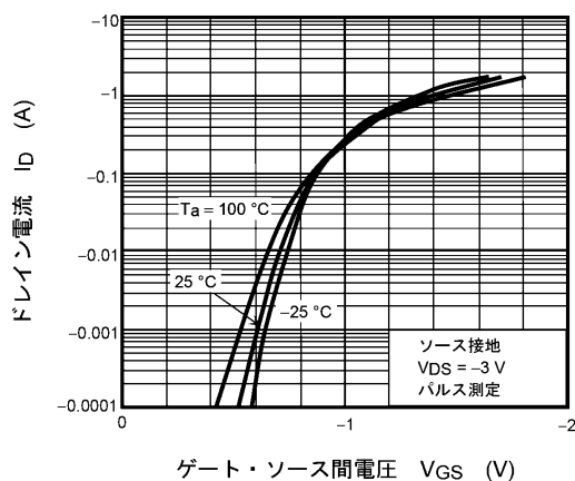
図 8.2 I_D - V_{GS}
