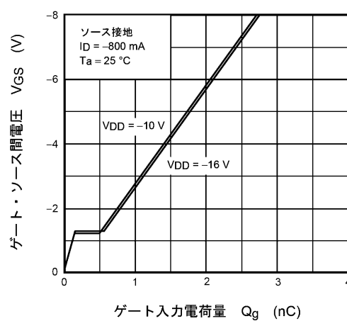
図 8.12 ダイナミック入力特性
