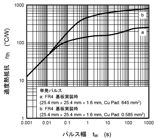
図 8.13 r_{th} - t_w
