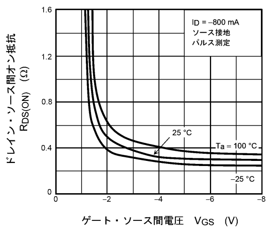
図 8.4 R_{DS(ON)} - V_{GS}
