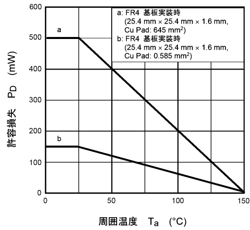
図 8.14 P_D - T_a
