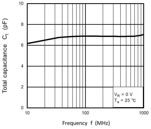
図 9.4 C_t - f
