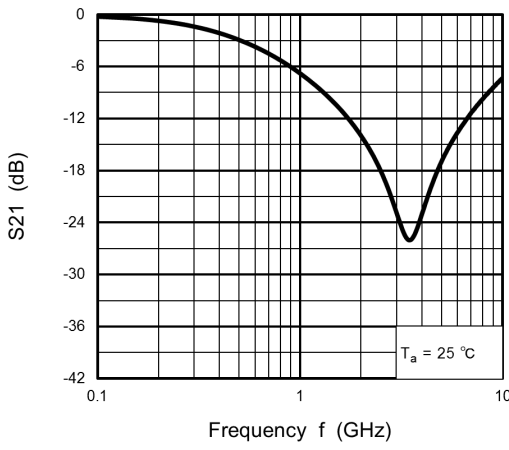
図 9.5 S_{21} - f
