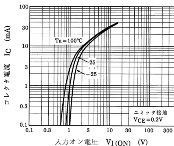
図 10.2 RN1908FE I_C - V_{I(ON)}
