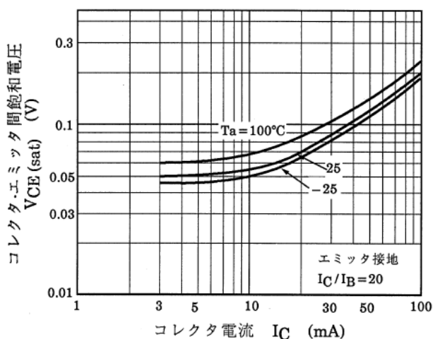
図 10.10 RN1907FE V_{CE(sat)}-I_C
