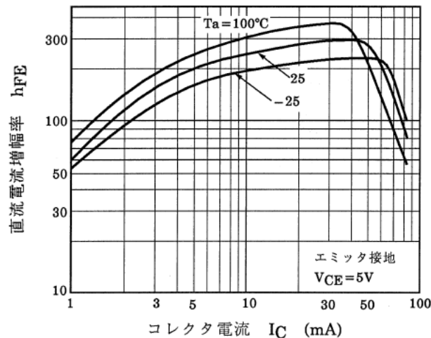
図 10.8 RN1908FE h_{FE}-I_C
