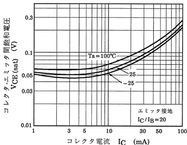
図 10.11 RN1908FE V_{CE(sat)}-I_C
