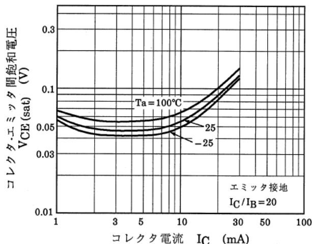
図 10.12 RN1909FE V_{CE(sat)}-I_C
