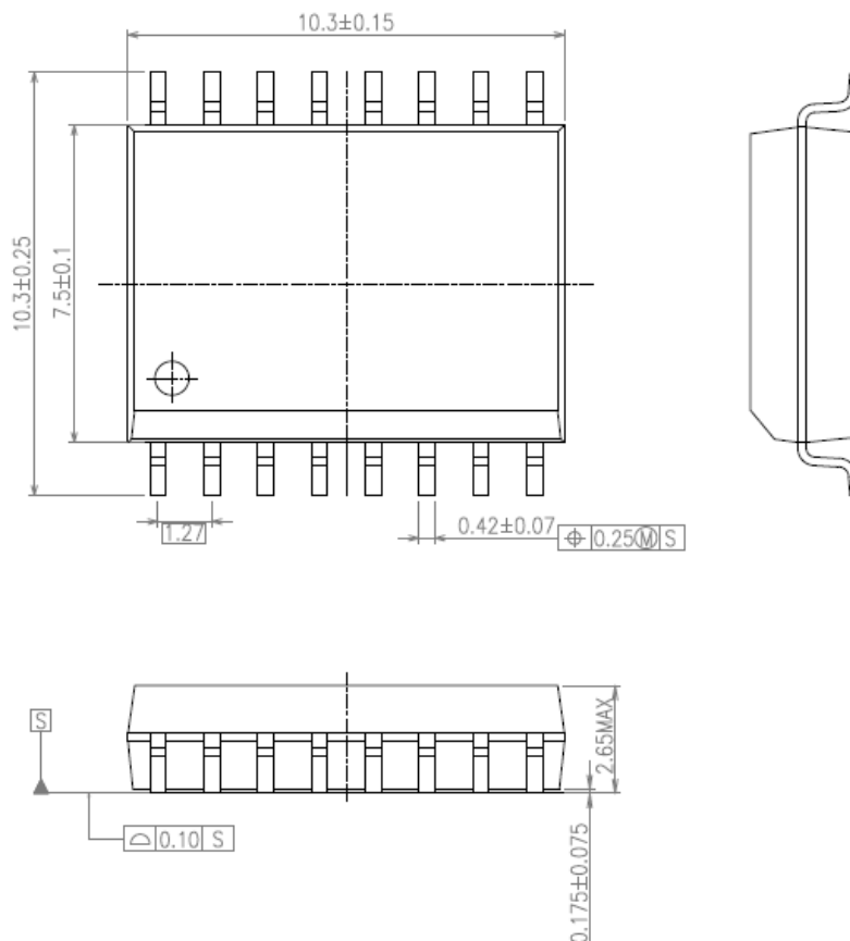
図 14.1 外形寸法図
