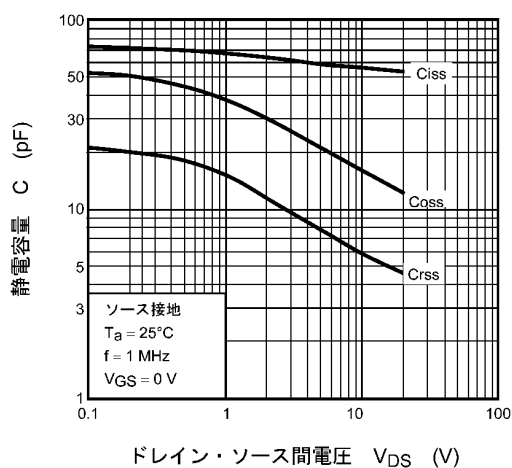
図 7.9 C - V_{DS}
