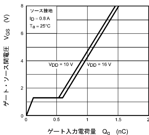
図 7.11 ダイナミック入力特性
