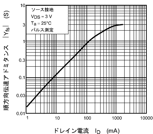
図 7.7 |Y_{fs}| - I_D
