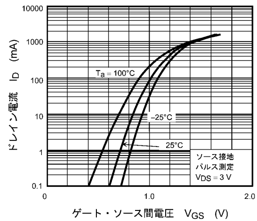
図 7.2 I_D - V_{GS}
