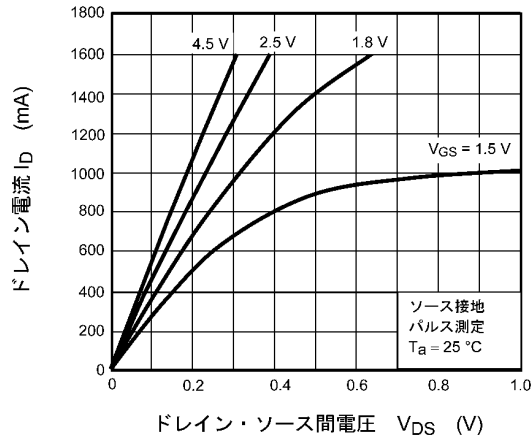
図 7.1 I_D - V_{DS}
