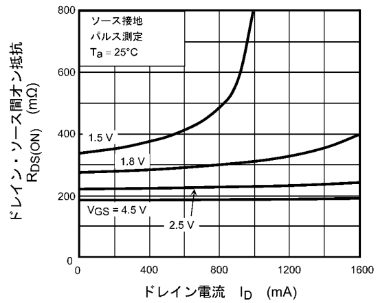
図 7.4 R_{DS(ON)} - I_D
