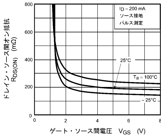
図 7.3 R_{DS(ON)} - V_{GS}
