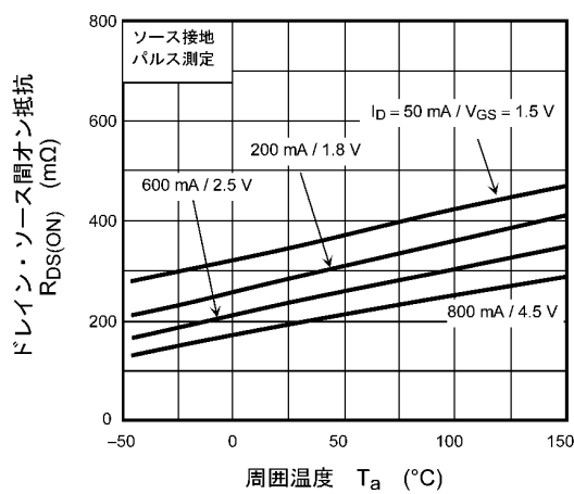
図 7.5 R_{DS(ON)} - T_a
