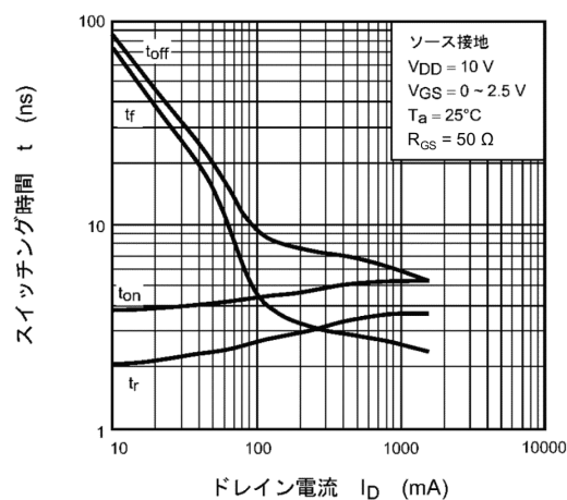
図 7.10 t - I_D
