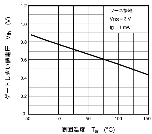
図 7.6 V_{th} - T_a
