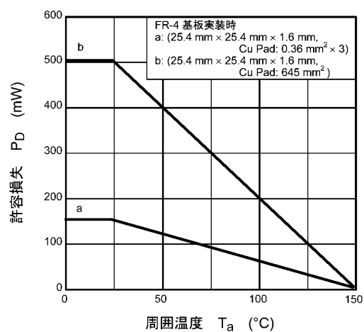
図 7.12 P_D - T_a
