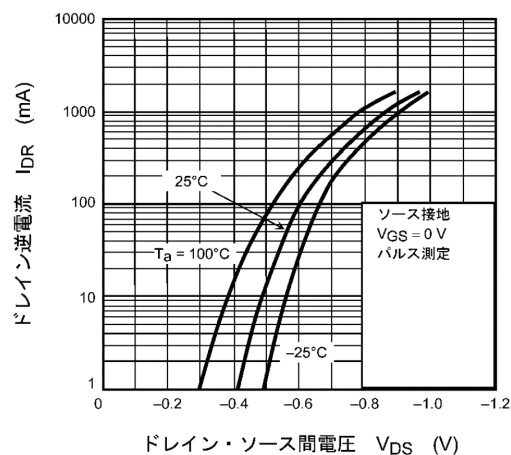
図 7.8 I_{DR} - V_{DS}
