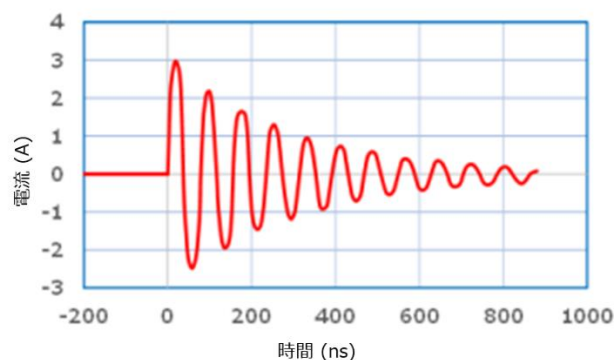
試験波形例 (ESD印加電圧イメージ)
