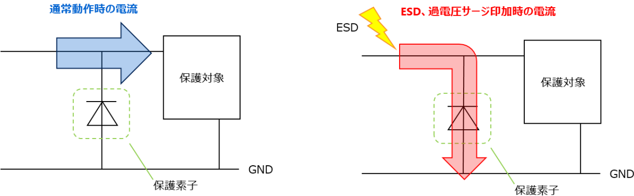
図 4.1 通常動作時とサージ印加時における保護素子の動作
