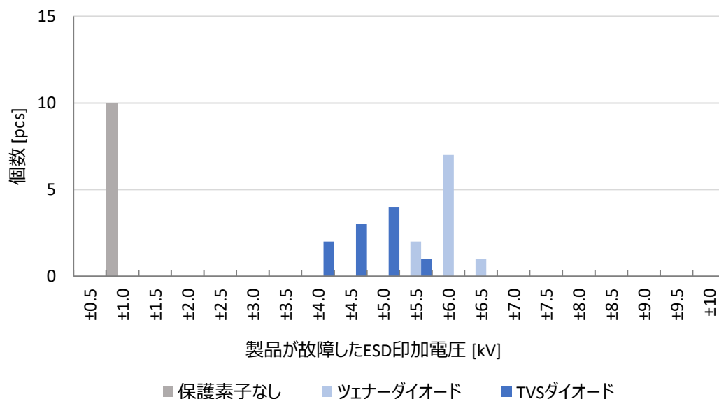
図 5.5 TLP172AM の ESD-HBM 試験結果
