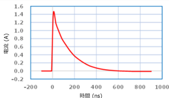
試験波形例 (ESD印加電圧イメージ)
