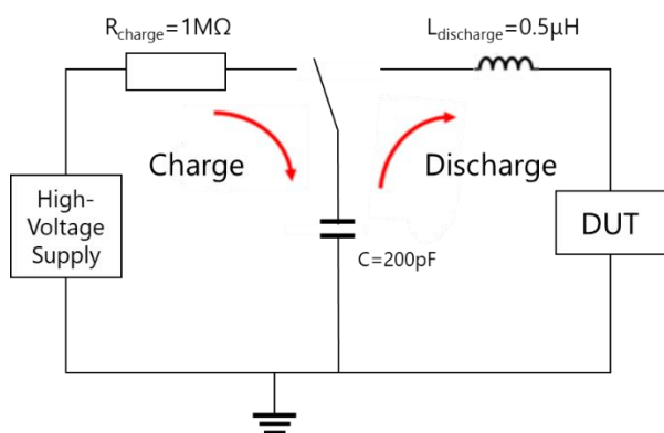
試験回路例
