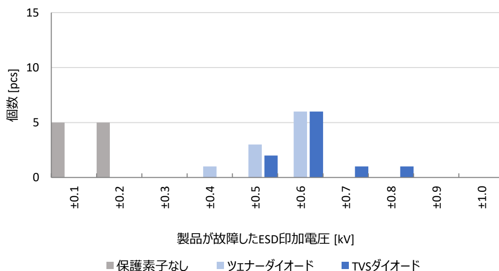
図 5.6 TLP172AM の ESD-MM 試験結果
