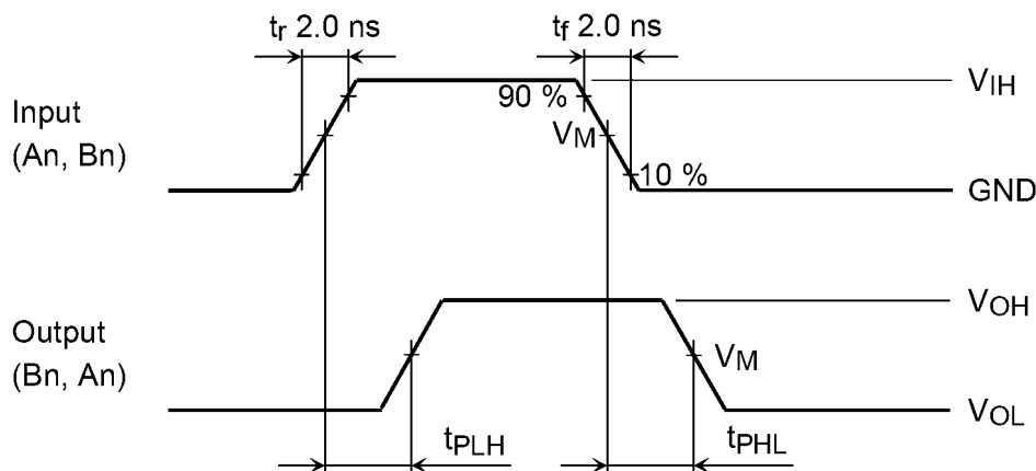
Fig. 13.1 t_{PLH} , t_{PHL}
