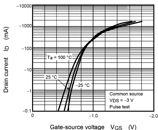
Fig. 7.2 I_D - V_{GS}
