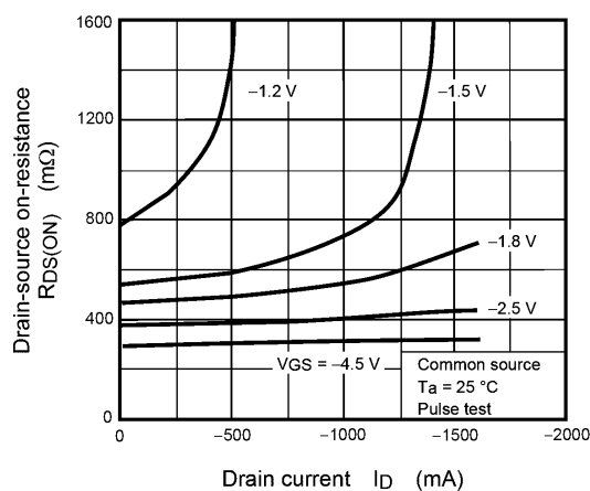
Fig. 7.6 R_{DS(ON)} - I_D
