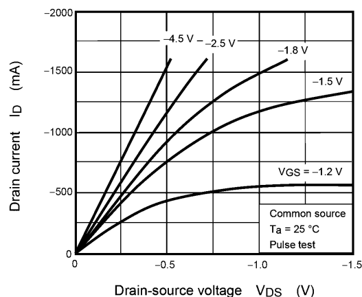
Fig. 7.1 I_D - V_{DS}
