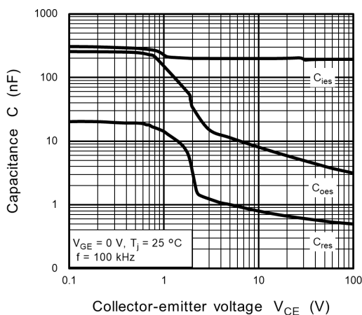
Fig. 7.4 Capacitance - V_{CE}
