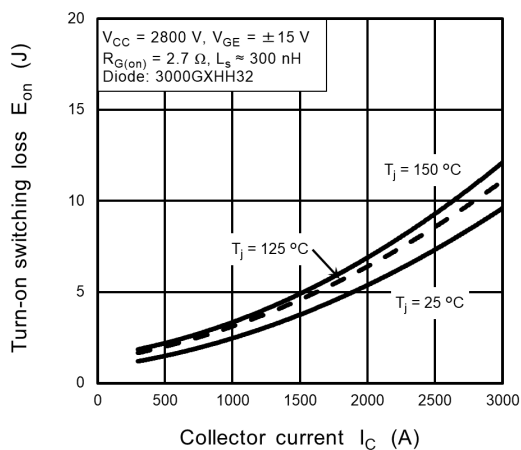
Fig. 7.5 E_{on} - I_C
