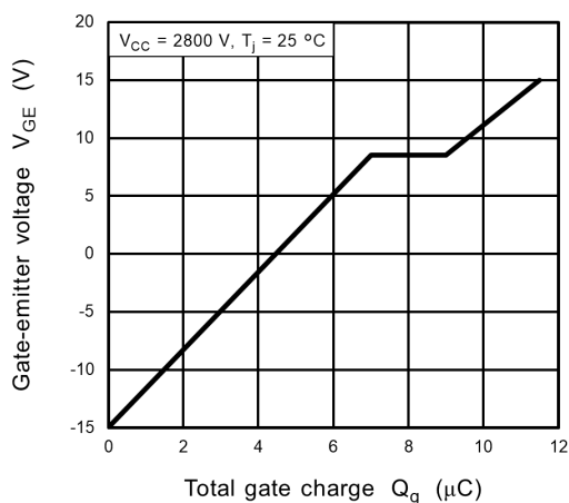
Fig. 7.3 V_{GE} - Q_g
