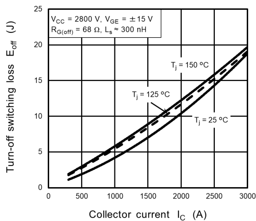
Fig. 7.6 E_{off} - I_C
