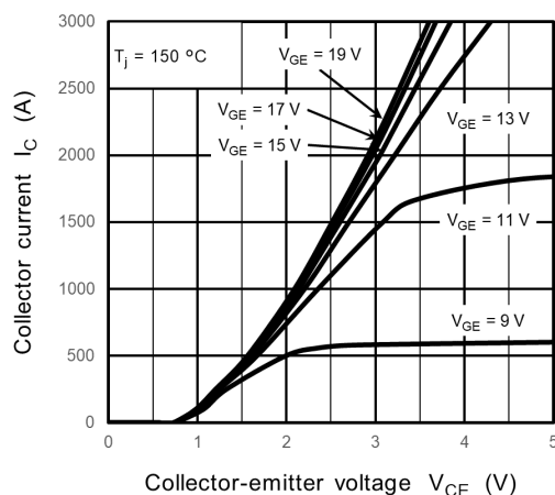
Fig. 7.2 I_C - V_{CE}
