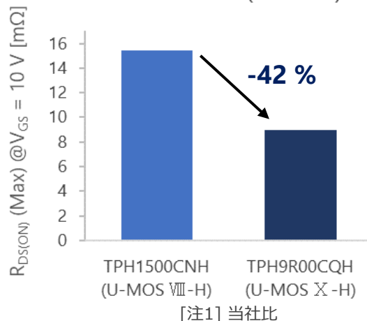
オン抵抗比較 (150 V品)
