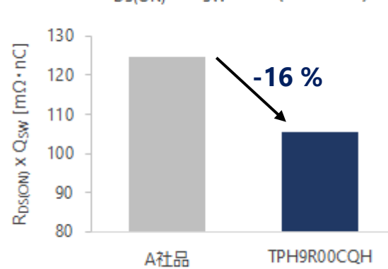
R_{DS(ON)} \times Q_{SW} 比較 (150 V品)
