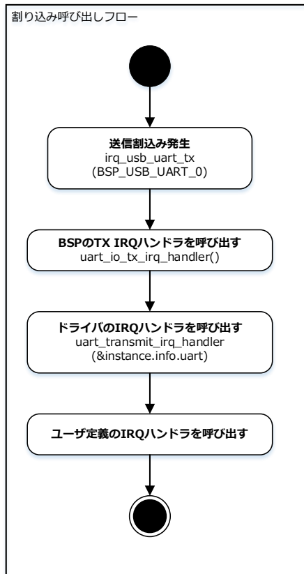
割り込み呼び出しフロー
