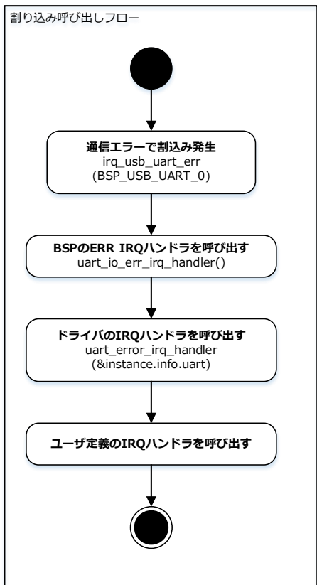
割り込み呼び出しフロー
