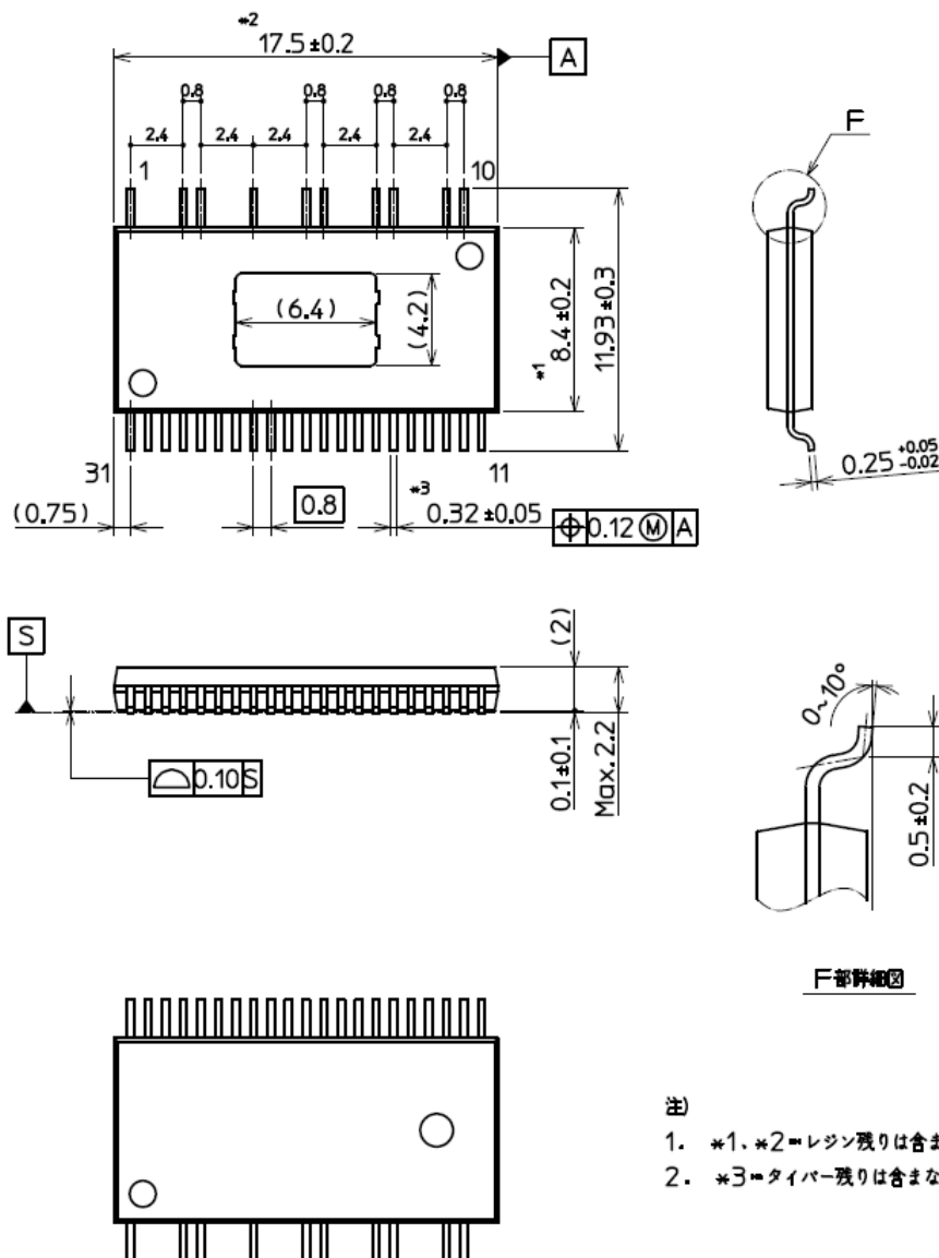
図 2.2.1 HSSOP31 パッケージ 外形寸法
