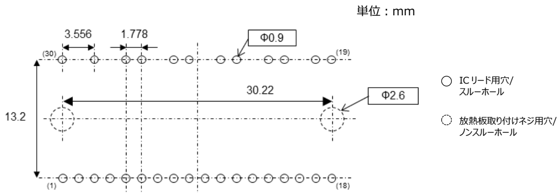
図 2.1.4 HDIP30 ランドパターン (参考)
