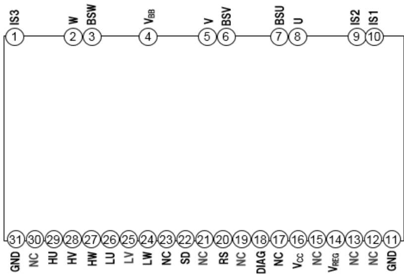
图 3.1.2 HSSOP31 端子配置图 (TPD4163F/TPD4164F)
