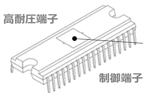
図 2.1.1 HDIP30 パッケージ
