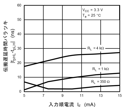
図 12.2.24 |t_{pHL} - t_{pLH}| - I_F
