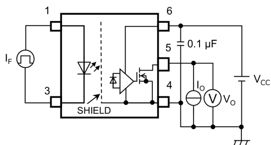
図 12.1.5 I_{FHL} , I_{FLH} , I_{HYS} 測定回路
