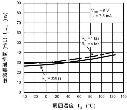
図 12.2.13 t_{pHL} - T_a
