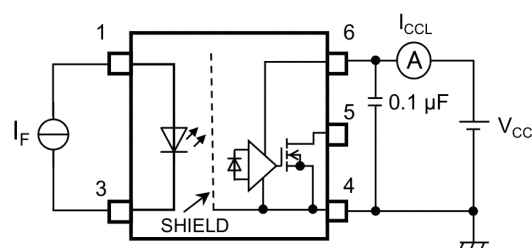
図 12.1.4 I_{CCL} 測定回路
