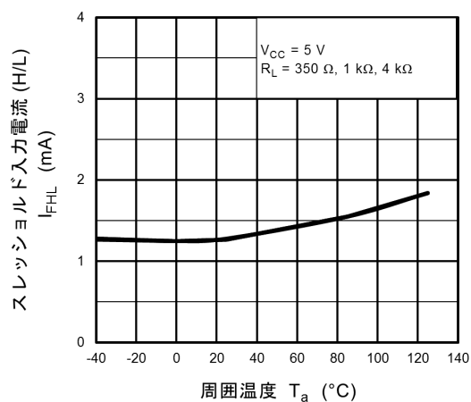
図 12.2.7 I_{FHL} - T_a
