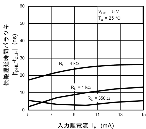
図 12.2.21 |t_{pHL} - t_{pLH}| - I_F
