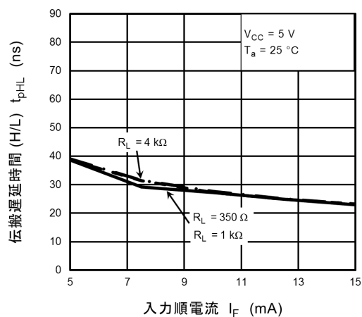
図 12.2.19 t_{pHL} - I_F
