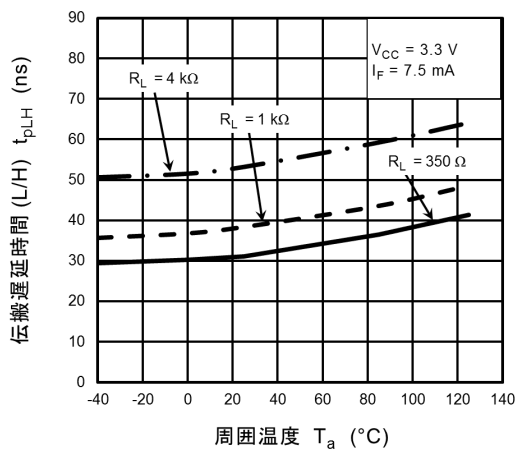
図 12.2.17 t_{pLH} - T_a
