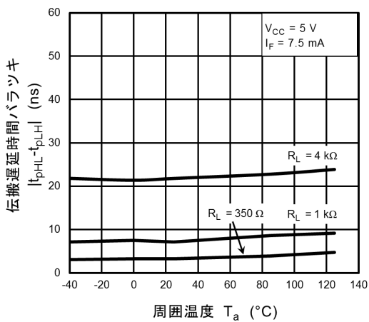
図 12.2.15 t_{pHL} - t_{pLH} - T_a
