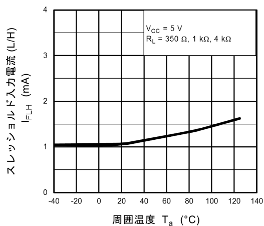
図 12.2.9 I_{FLH} - T_a
