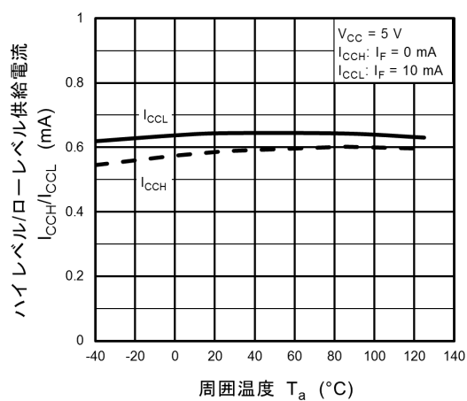
図 12.2.11 I_{CCH}, I_{CCL} - T_a
