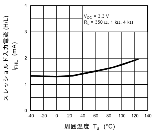
図 12.2.8 I_{FHL} - T_a
