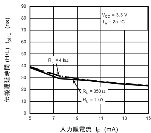
図 12.2.22 t_{pHL} - I_F
