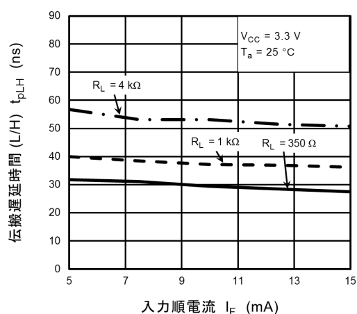
図 12.2.23 t_{pLH} - I_F
