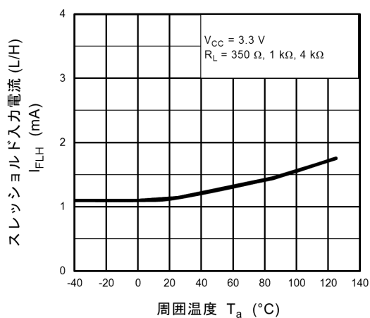
図 12.2.10 I_{FLH} - T_a
