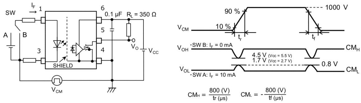
図 12.1.7 コモンモード過渡耐性測定回路, 波形
