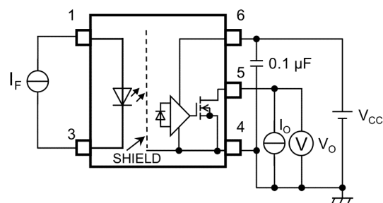
図 12.1.2 V_{OL} 測定回路
