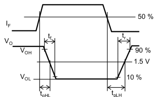
図 12.1.6 伝搬遅延時間測定回路, 波形
