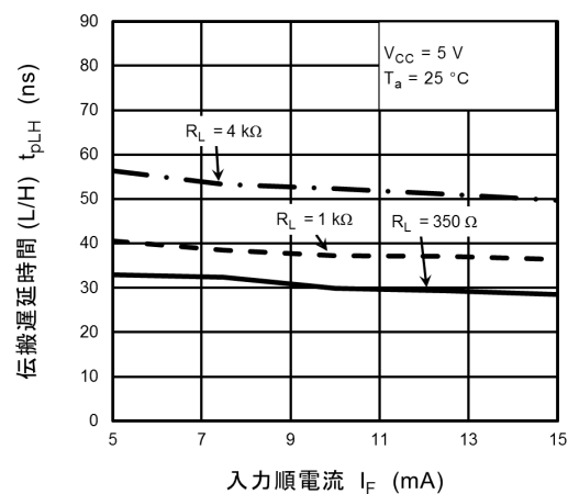
図 12.2.20 t_{pLH} - I_F
