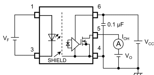
図 12.1.1 I_{OH} 測定回路
