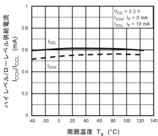
図 12.2.12 I_{CCH}, I_{CCL} - T_a
