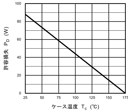
図 9.8 P_D - T_c (最大値 (保証値))
