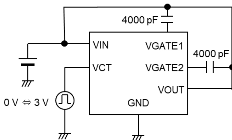
図 4 V_{GS} オン時間、オフ時間測定回路
