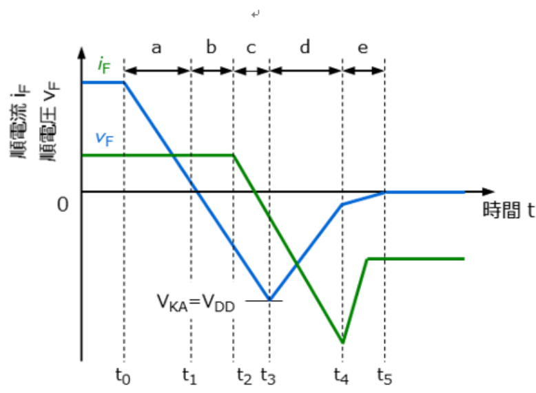
図 2.6 逆回復動作
