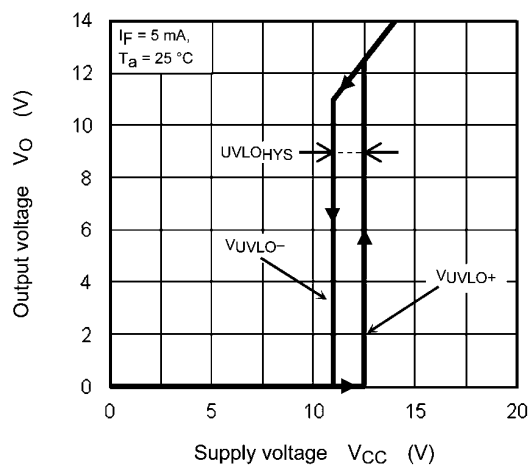
Fig. 13.2.11 V_O(V_{UVLO}) - V_{CC}
