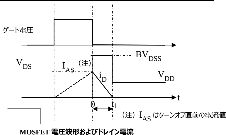
図 1.5 アバランシェ降伏時各部の波形
