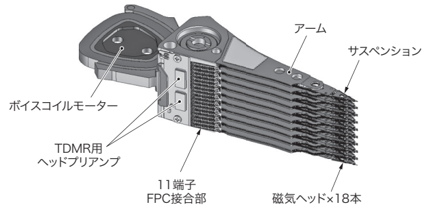
図2. 開発したTDMR用アクチュエーター
