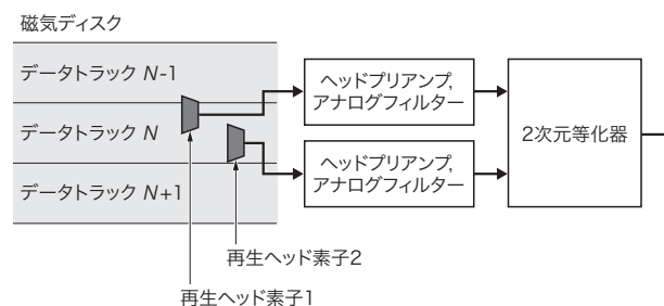
図4. TDMRによるデータ再生のイメージ
