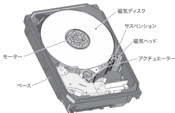
図1. MG08シリーズの内部構造
