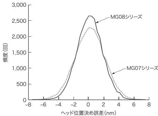
図5. ヘッド位置決め精度の比較
