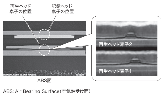
図3. TDMR用ヘッド素子部の走査型電子顕微鏡 (SEM) 像
