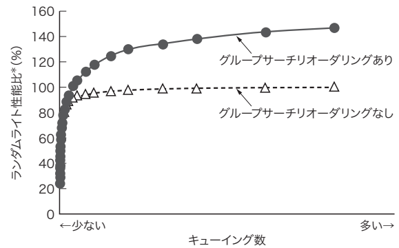
図6. ランダムライト性能の評価結果
