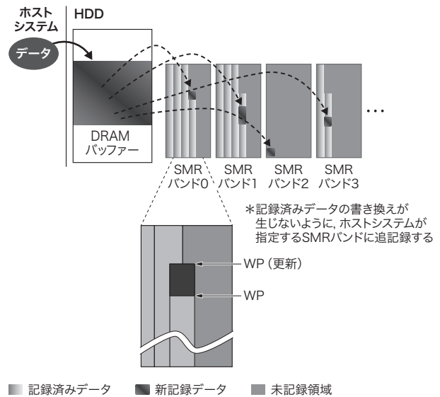
図6. HMタイプのランダムライト動作
