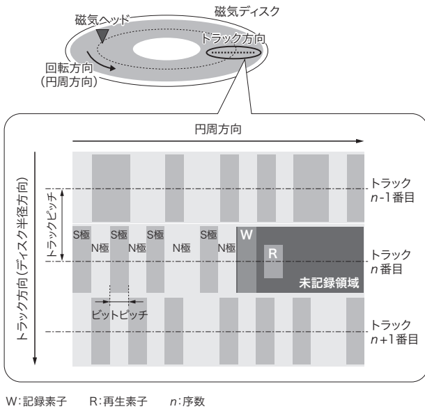
図1. HDDを構成する磁気ディスクと磁気ヘッドの概要
