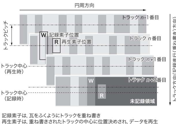
図2. SMR方式のトラックと、記録ヘッド、再生ヘッドの概略
