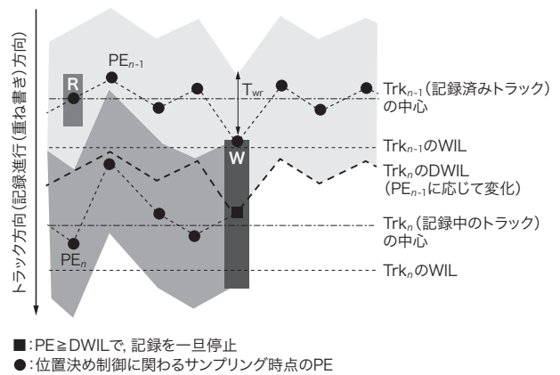
図9. DWILを適用したSMR HDDのデータ記録
