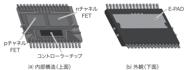
図5. TB9111FNGの内部構造と外観
