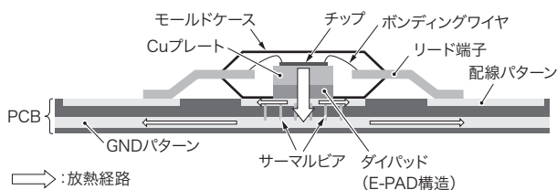
図4. PCBに実装されたパッケージと放熱経路の断面図
