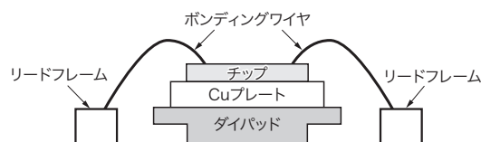
図2. TB9051FTGのパッケージ構造
